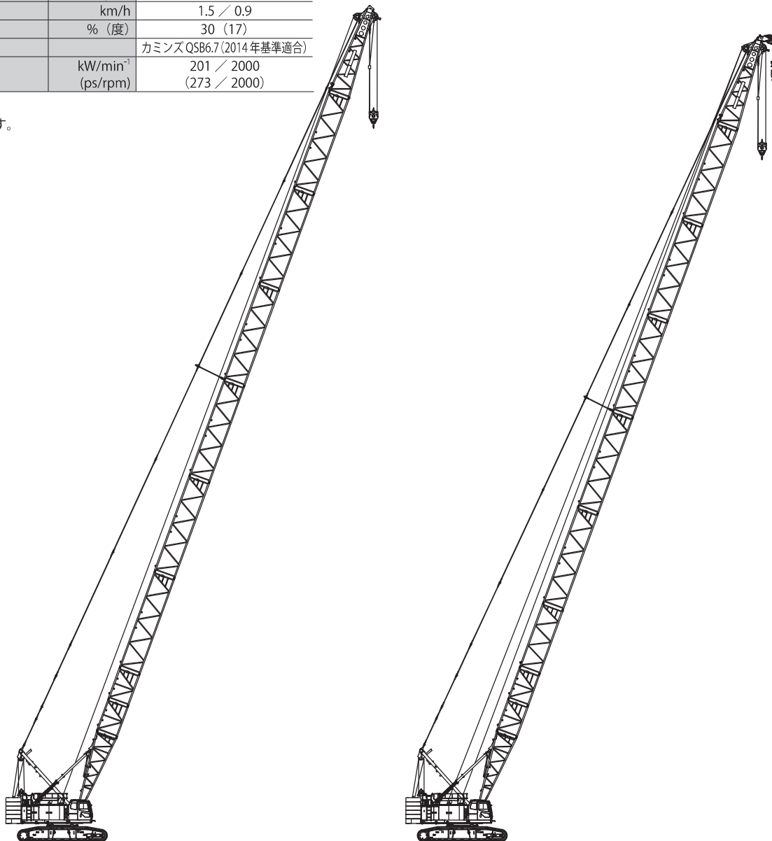
クレーン仕様 補助シーブ付きブーム最長
